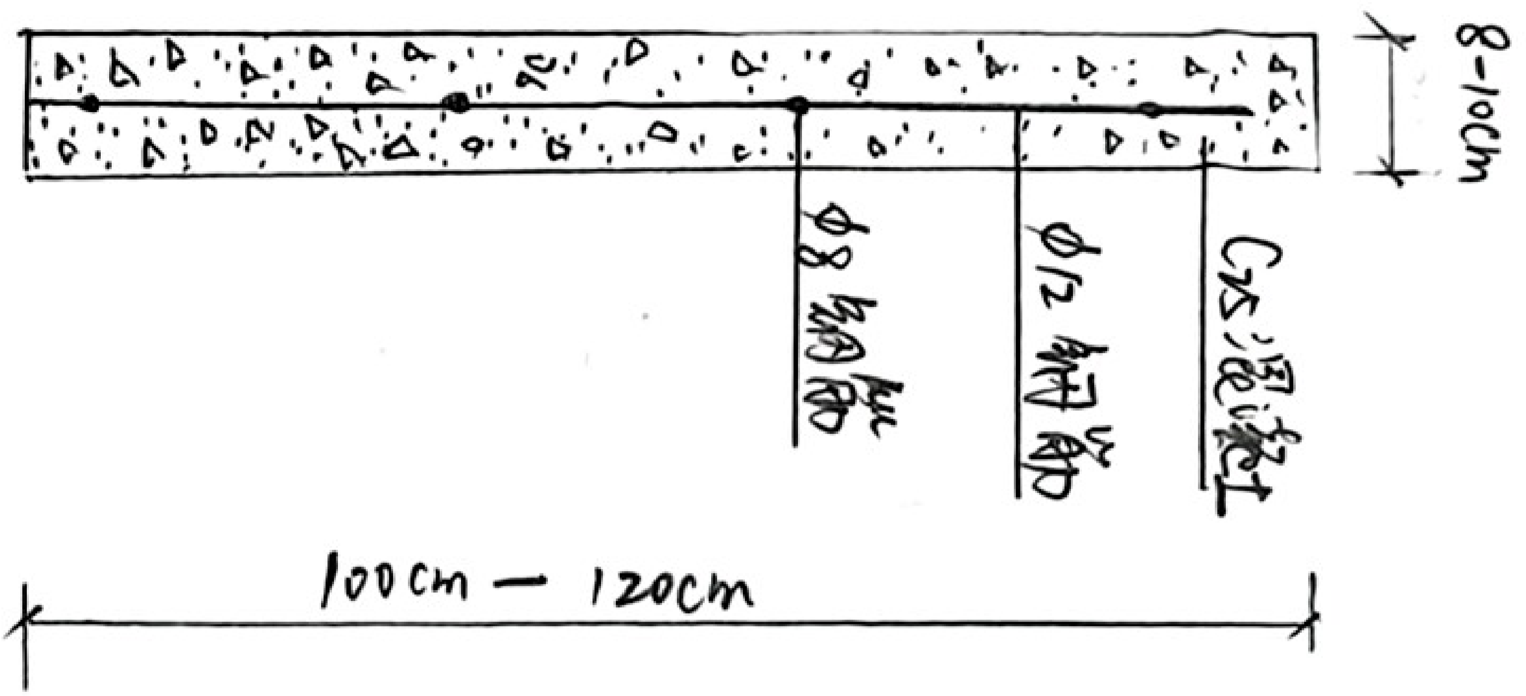
栏杆剖面图
