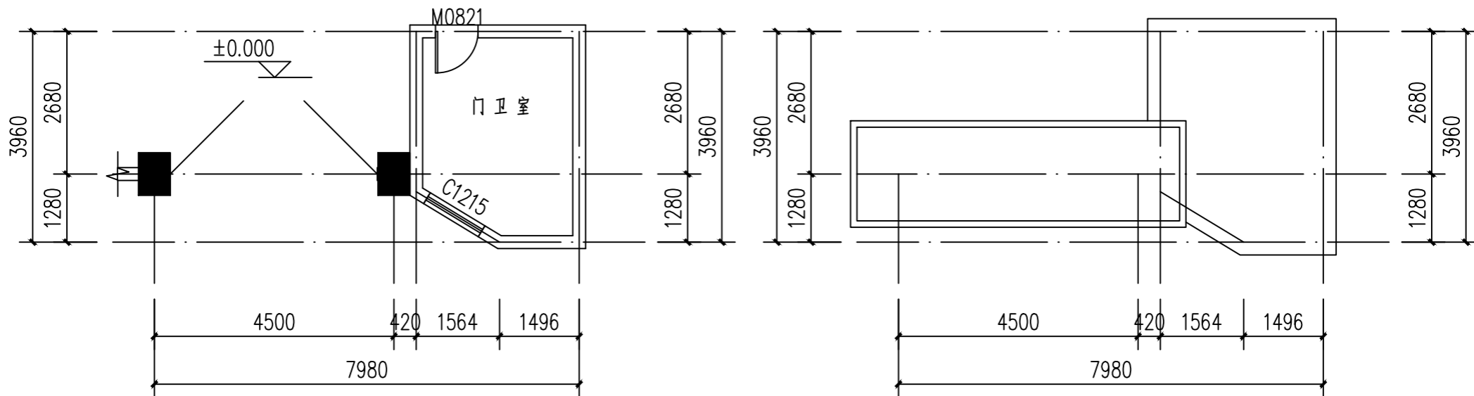
门楼平面图 1:100
