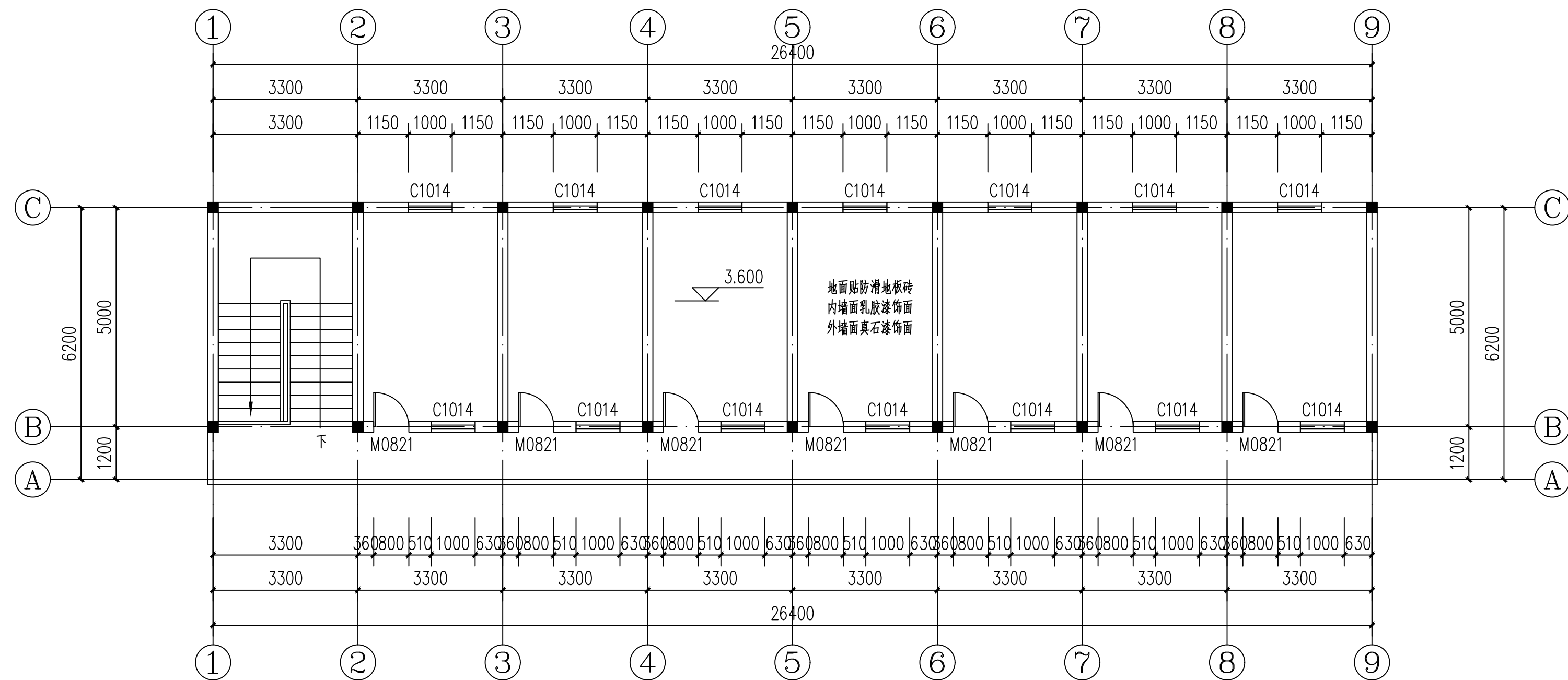
照料中心二层平面图 1:100
