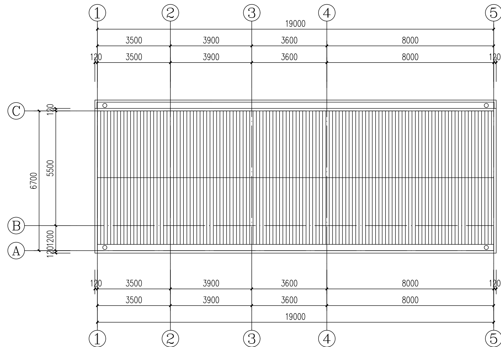
食堂屋面平面图 1:100
