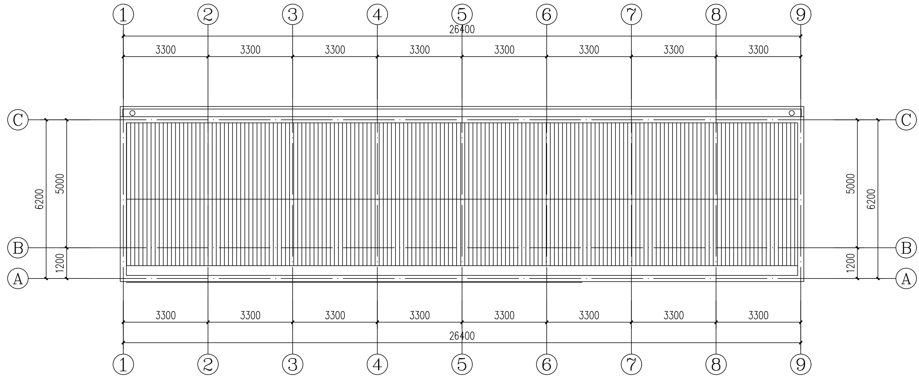
照料中心屋面平面图 1:100
