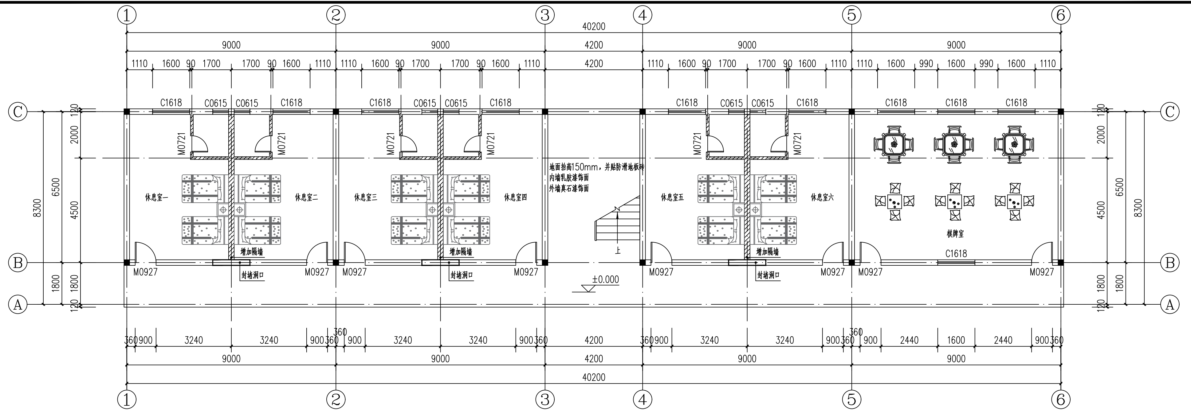
养老服务综合体一层平面图 1:100
