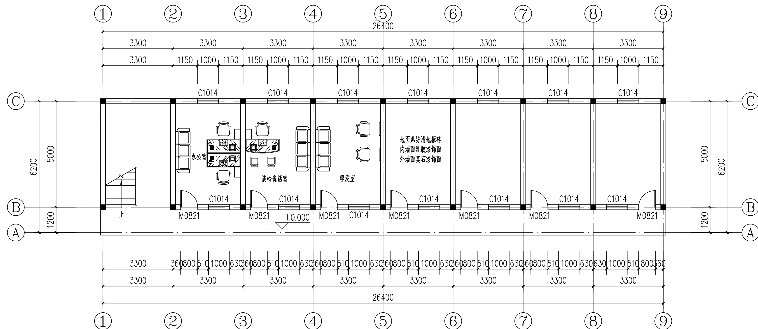
照料中心一层平面图 1:100
