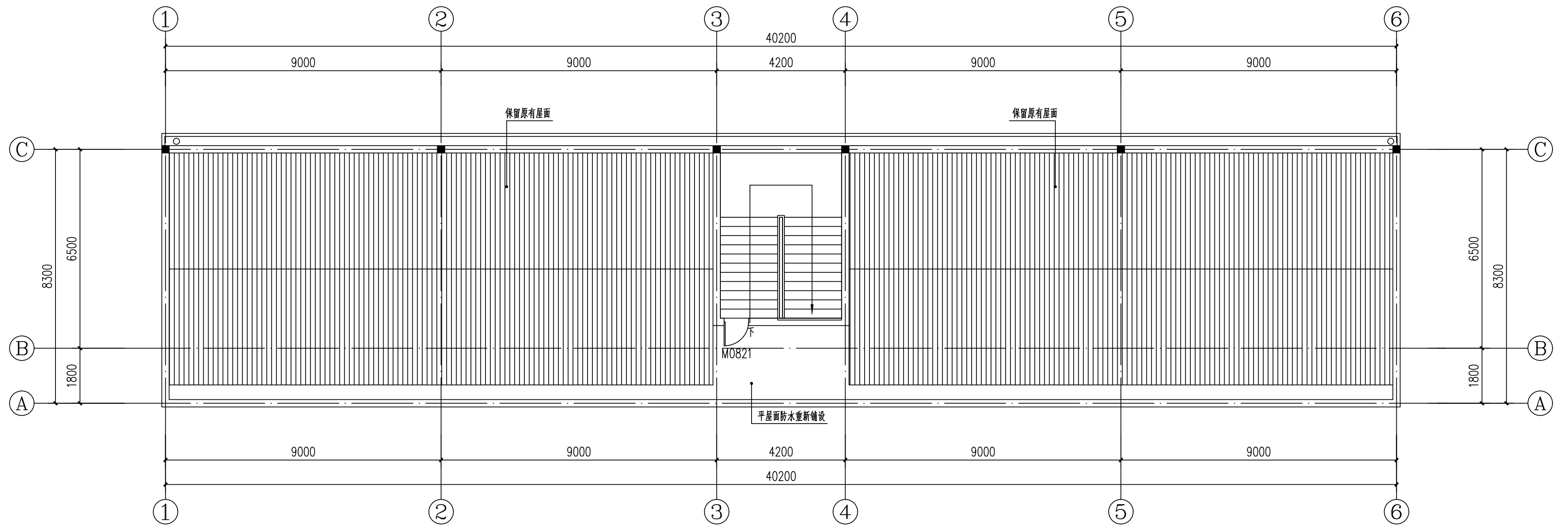
养老服务综合体屋面平面图 1:100
