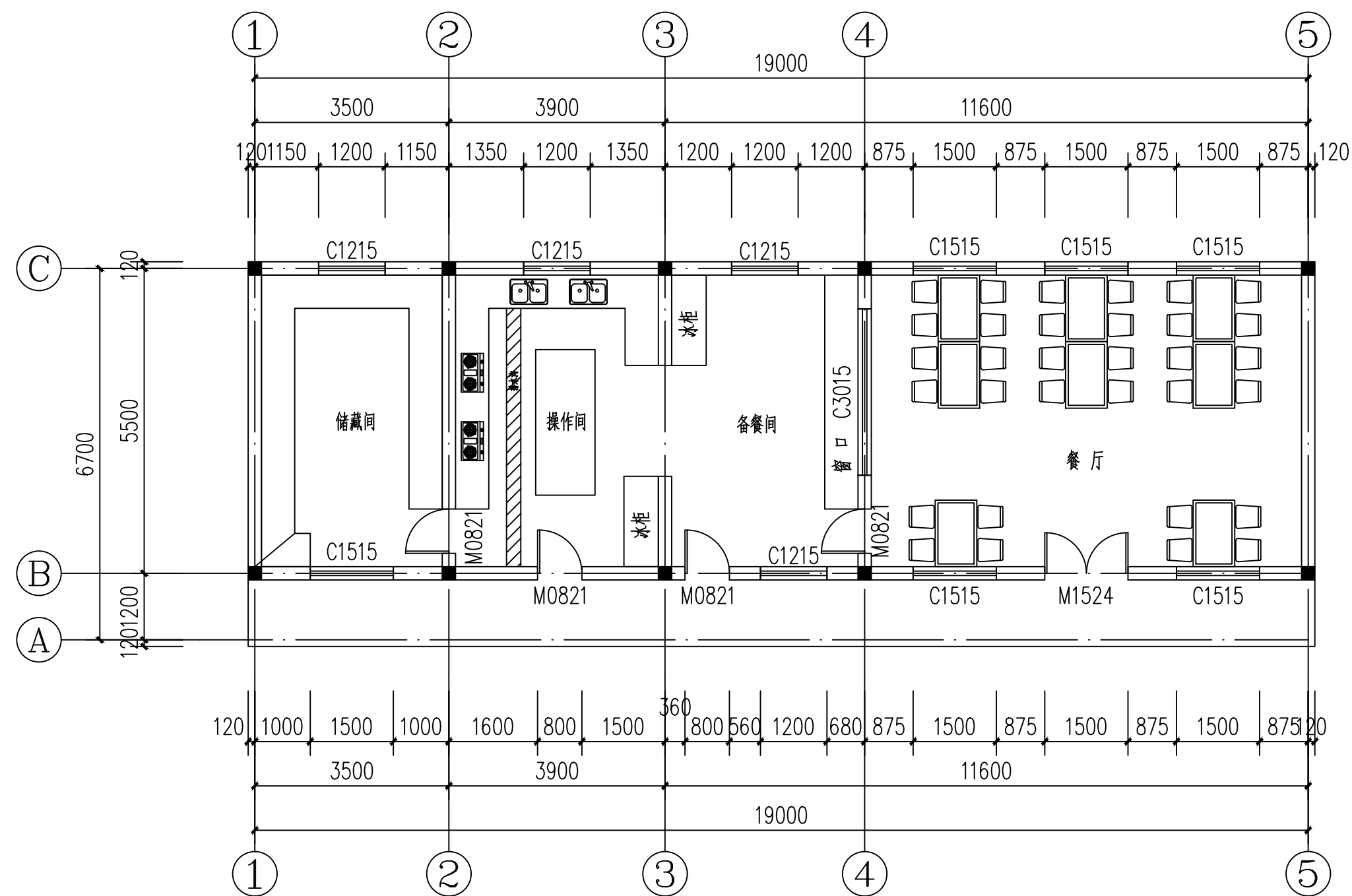
食堂平面图 1:100
