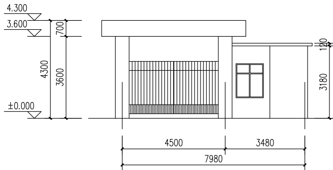
门楼正立面图 1:100
