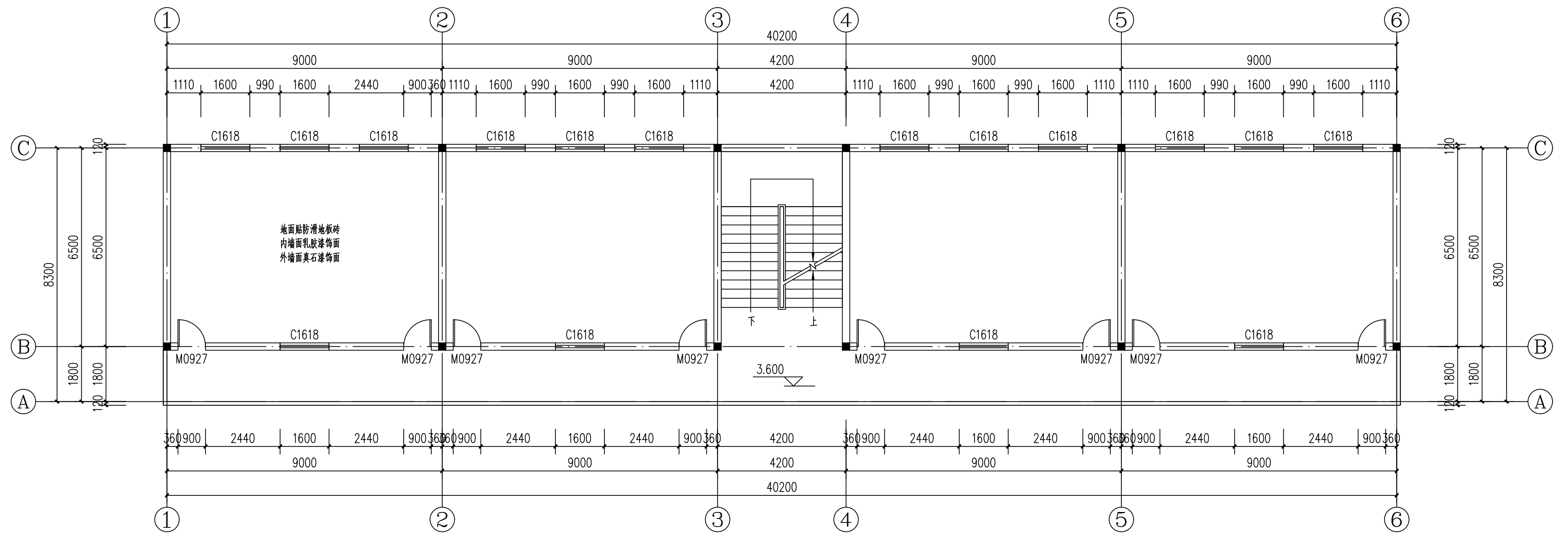
养老服务综合体二层平面图 1:100
