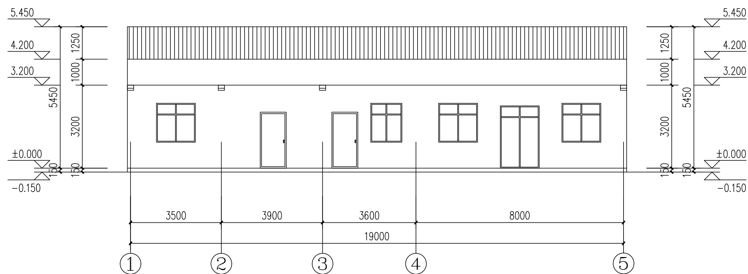
食堂正立面图 1:100
