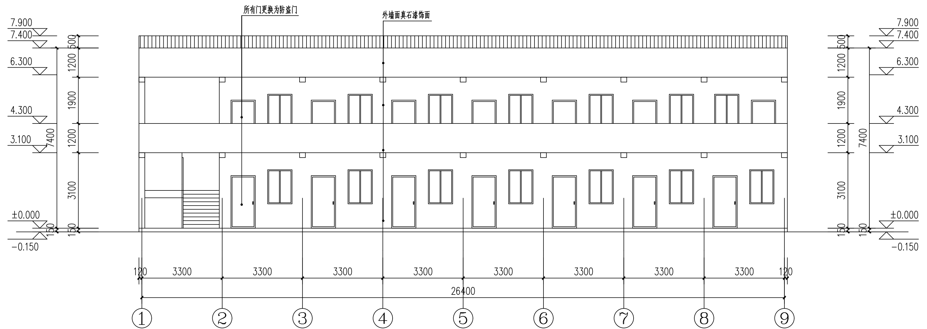
照料中心正立面图 1:100
