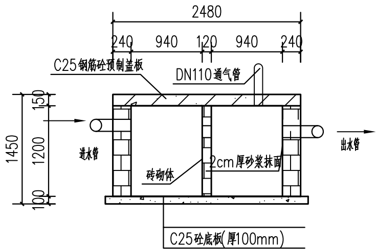
2m³化粪池剖面图 1:100
