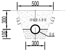
DN110PVC管开挖断面图
