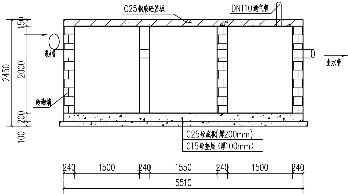
20m 3 化粪池剖面图 1:100
