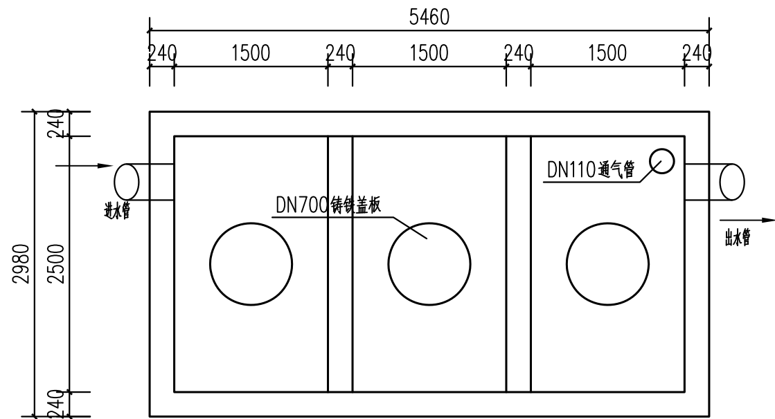
20m 3 化粪池平面图 1:100
