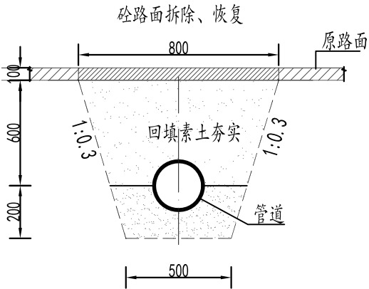
DN300波纹管开挖断面图(一)
