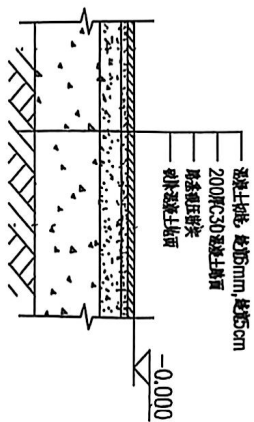
门口塘硬化剖面图
