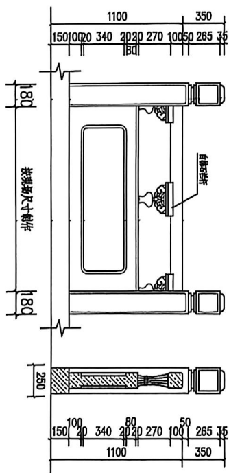
白楠石栏杆大样图
