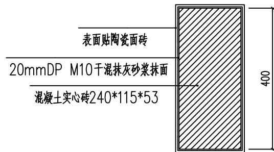
花池剖面图 1:100 说明: 花池总长: 90m
