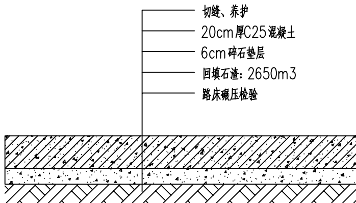
硬化路面剖面图 1:100 说明: 硬化总面积: 2650m 2
