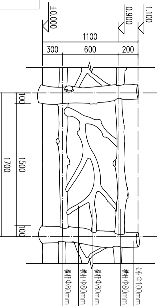
仿树藤栏杆详图 1:25
