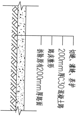
五组混凝土地面大样图—1:25
