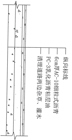
五组道路刷黑剖面图 1:50
