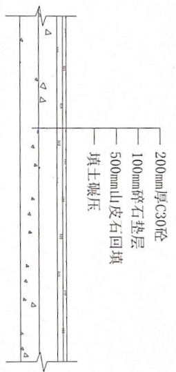
剖面图 1:50
