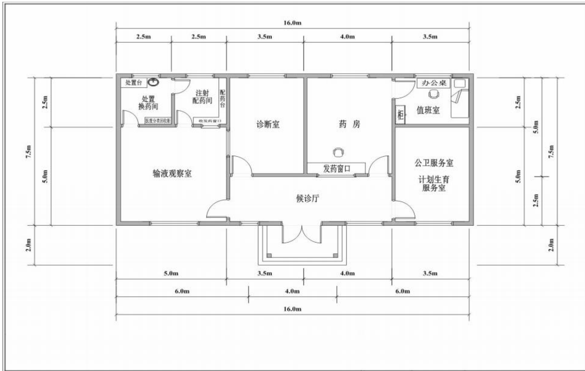
图例 1: 湖北省村卫生室科室布局平面示意图 (建筑面积: 120 m 2 )
